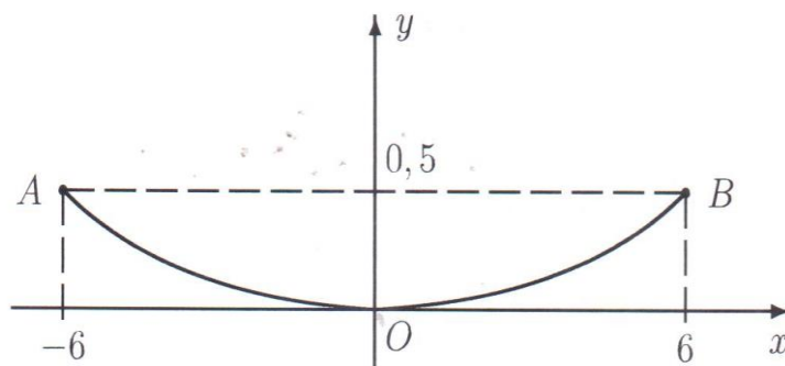
Рисунок 28 – Эскиз параболы
