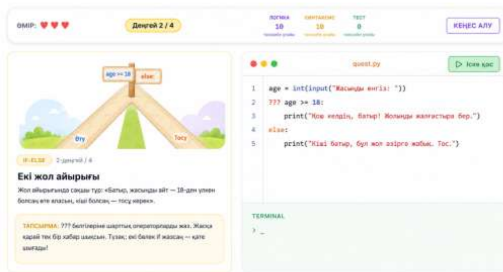
Сурет 34 – екінші деңгей: «Екі жол айырығы» тапсырмасы
